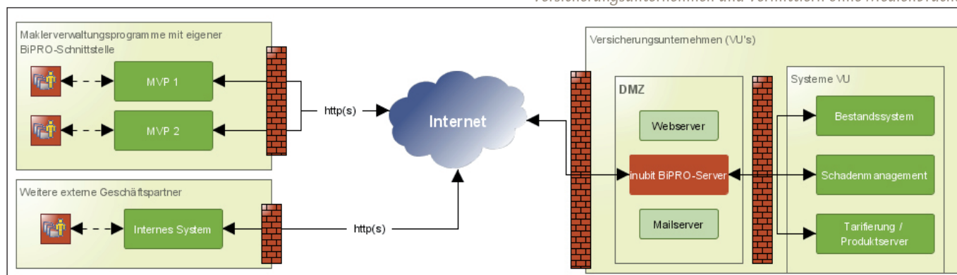
Der inubit BiPRO-Server steuert Prozesse zwischen Versicherungsunternehmen und Vermittlern ohne Medienbrüche.
